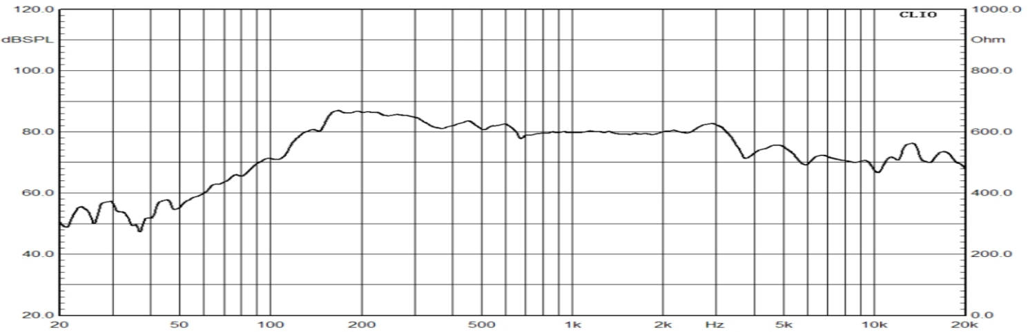
SPL
