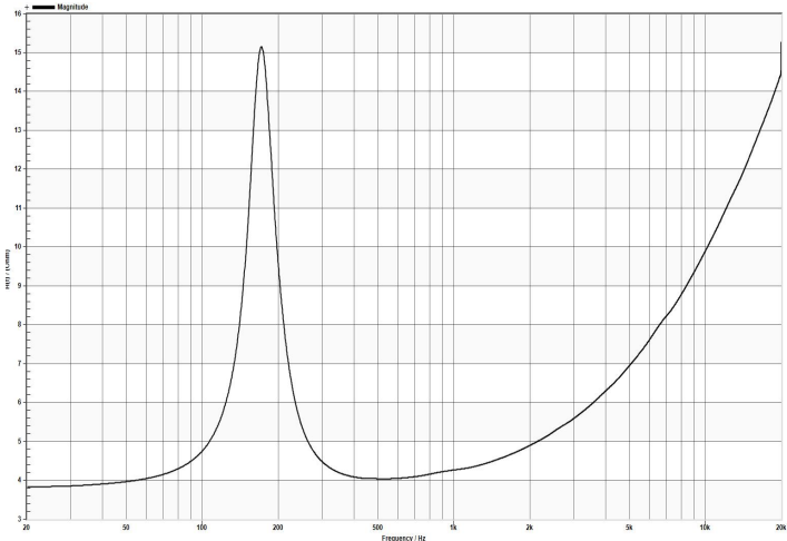
IMP
