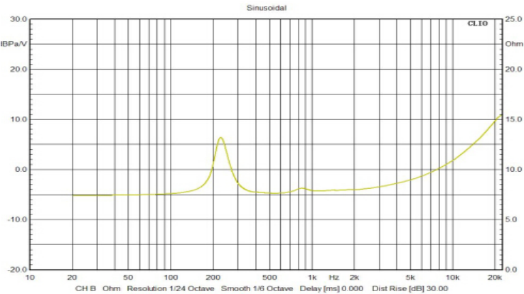
IMP
