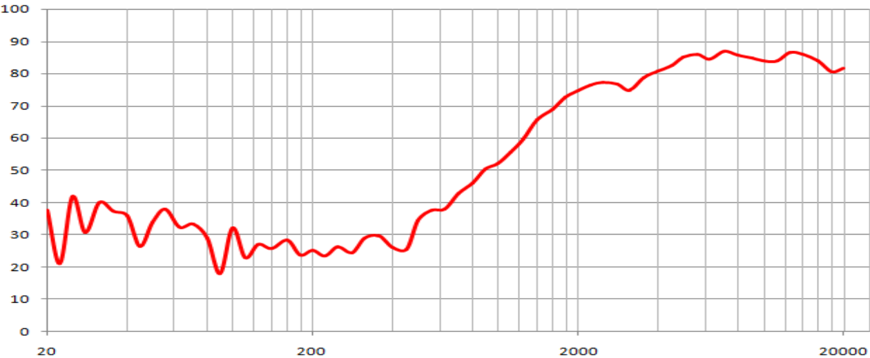
SPL
