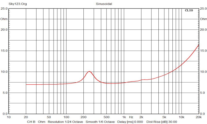
IMP
