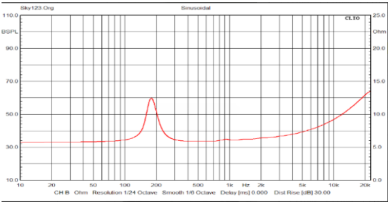
IMP
