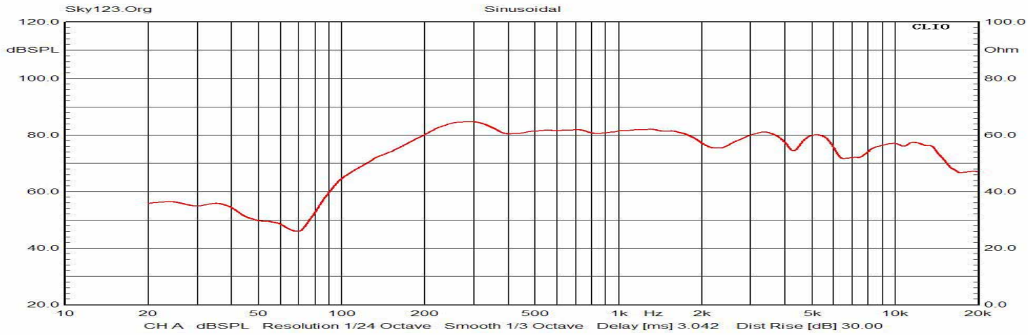
SPL
