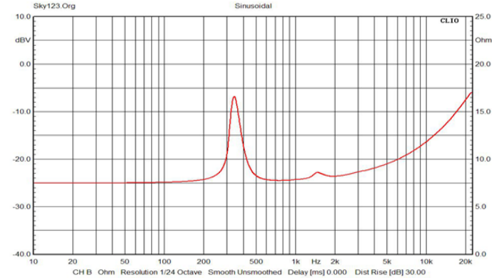
IMP
