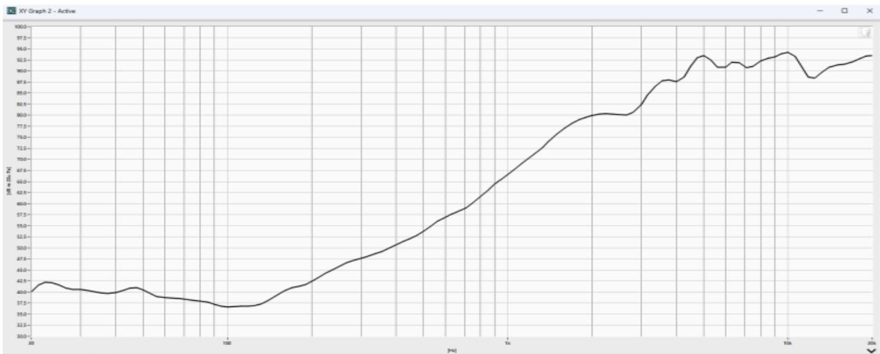
SPL
