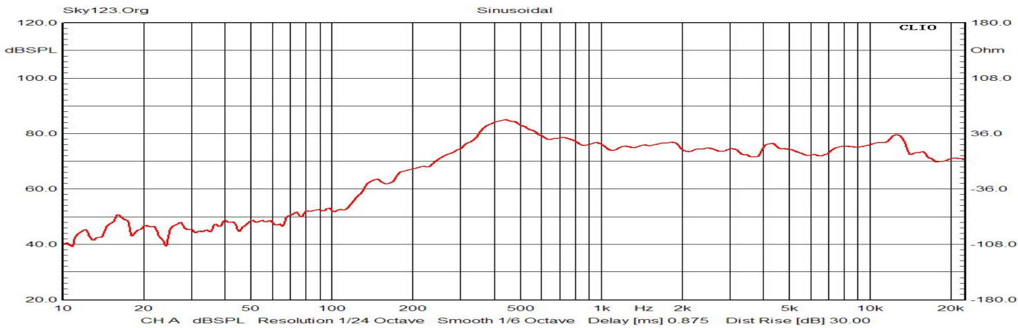
SPL
