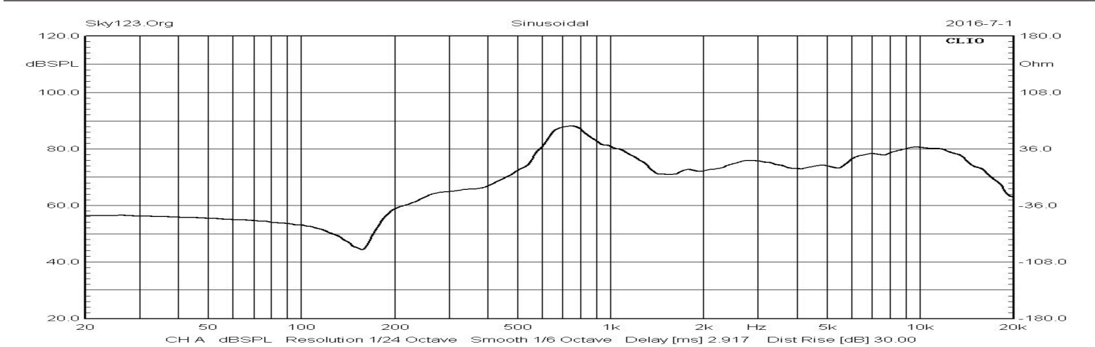
SPL
