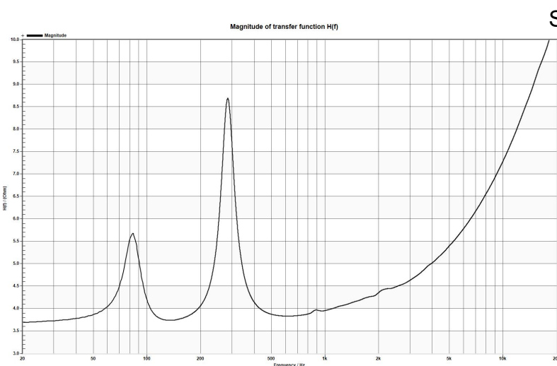
IMP
