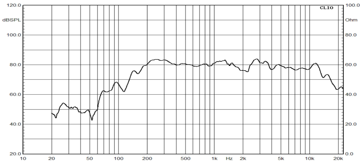
SPL
