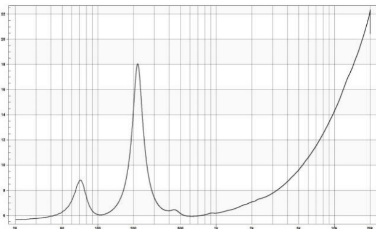
IMP
