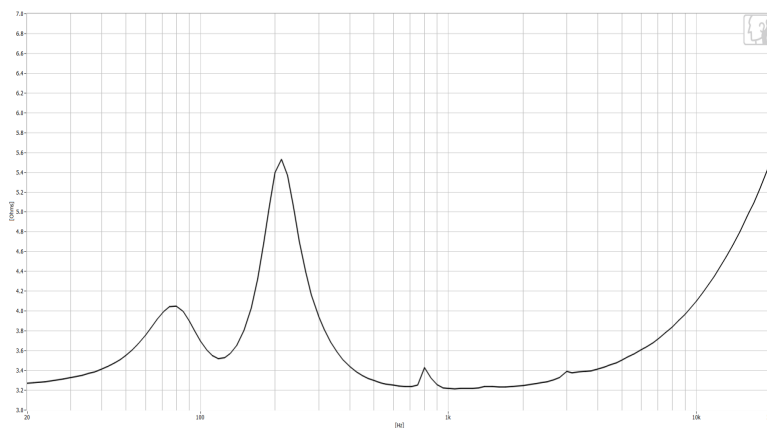
IMP
