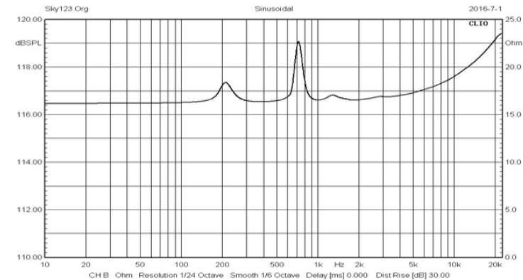
IMP
