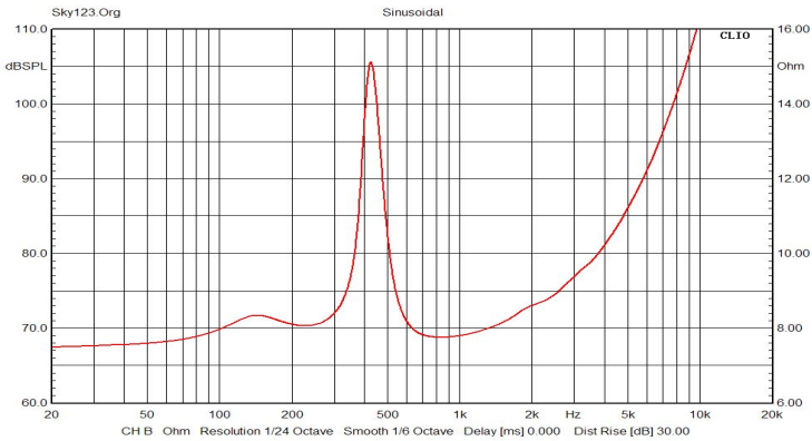
IMP
