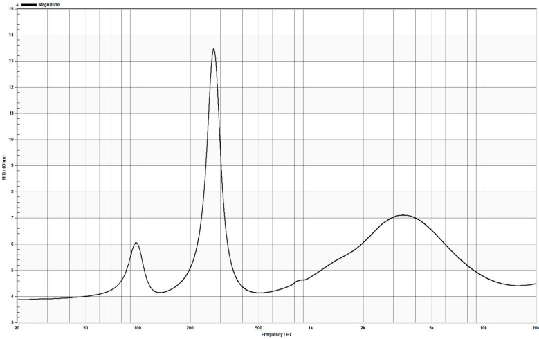
IMP
