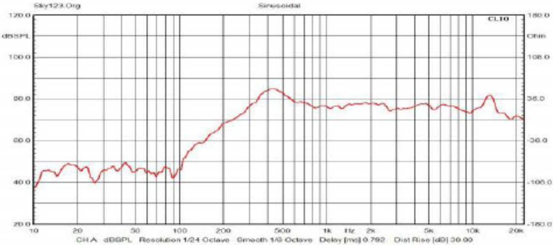
SPL
