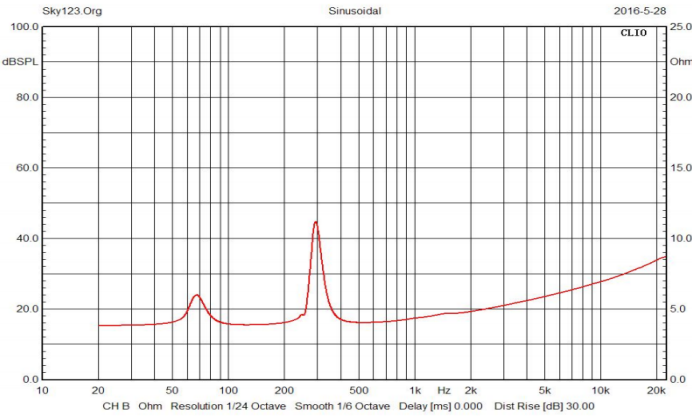
IMP
