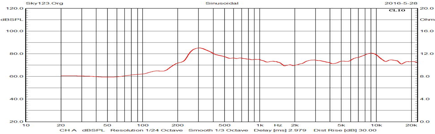
SPL
