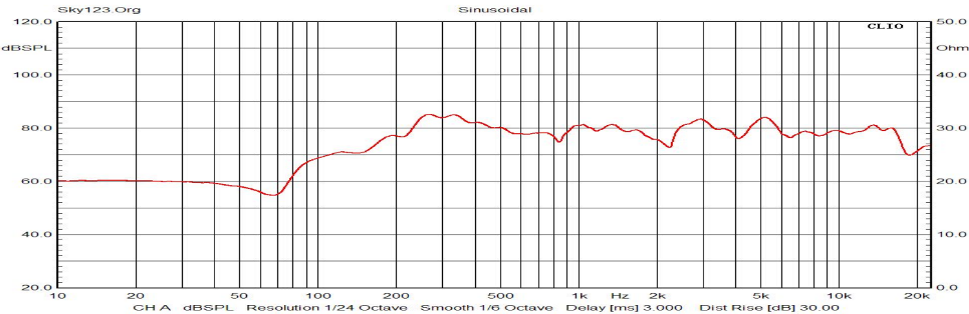
SPL
